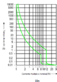
Curva D
