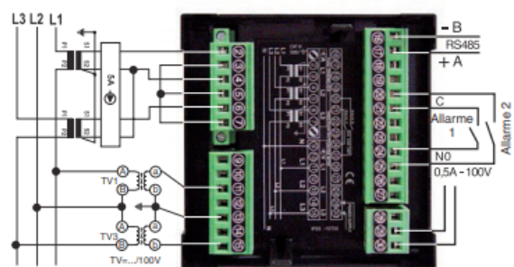
2RAE96L4CS485H2 2RAE96L4CS485H3 Inserción ARON
