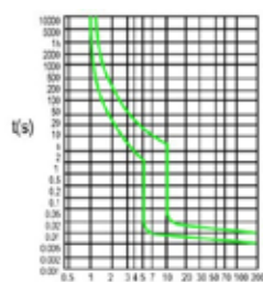
Curva C
