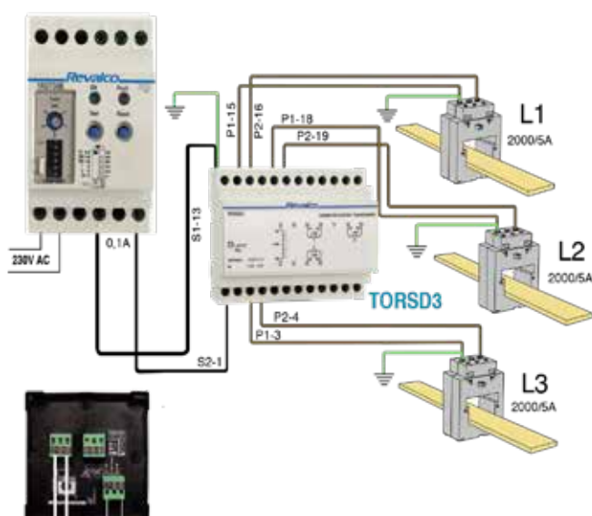
TORSD3 5+5+5A/0,1A con transformador de intensidad clase 0,2 LINEA SIN NEUTRO
