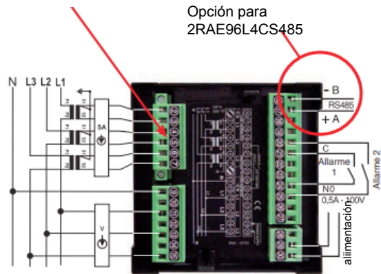
2RAE96L4CS inserción con neutro
