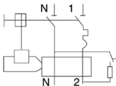
Diagrama de cableado
