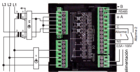
2RAE96L4CS485H1 Inserción ARON
