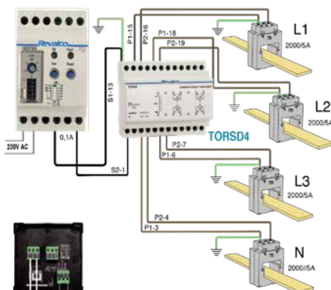
TORSD4 5+5+5+5A/0,1A con transformador de intensidad clase 0,2 LINEA CON NEUTRO
