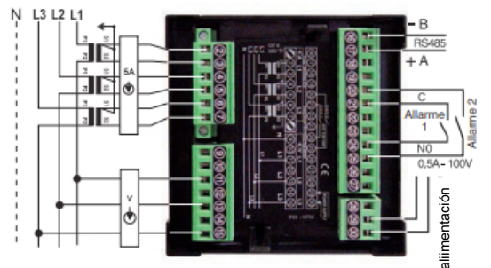
2RAE96L4CS485H1 inserción sin neutro
