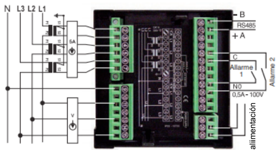
2RAE96L4CS485H1 inserción con neutro
