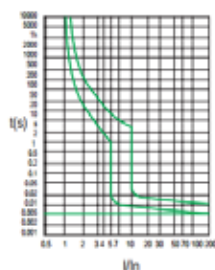
Curva C
